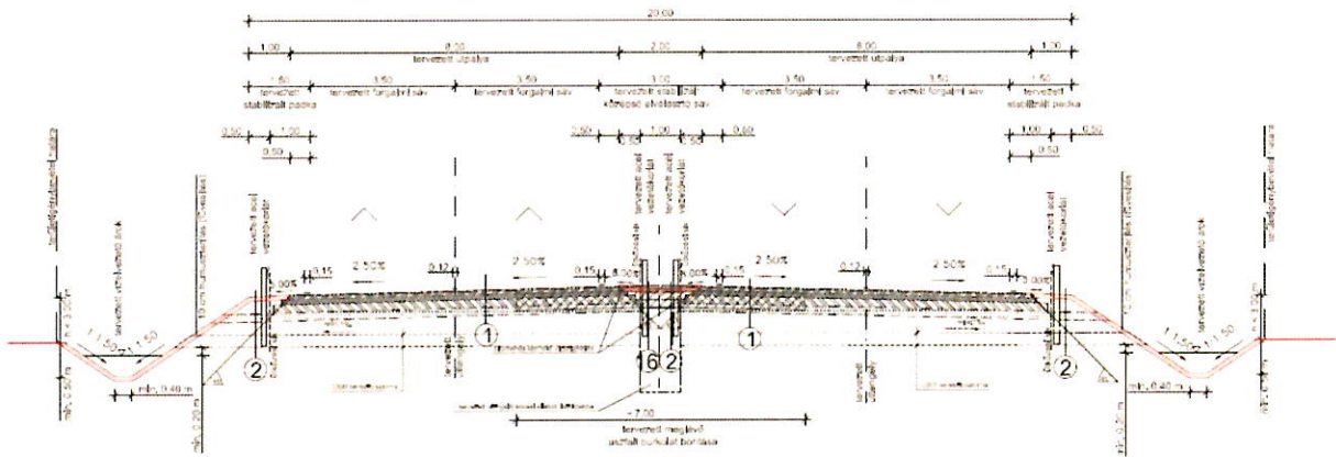
MKSZ. 7. MINTAKERESZTSZELVÉNY 7. 57 sz. főút, tervezett 2x2 sávossal burkolatú út (23+423,77 - 24+347,63 km szelvények között) Töltésmagasság < 3m v h =90km/h
